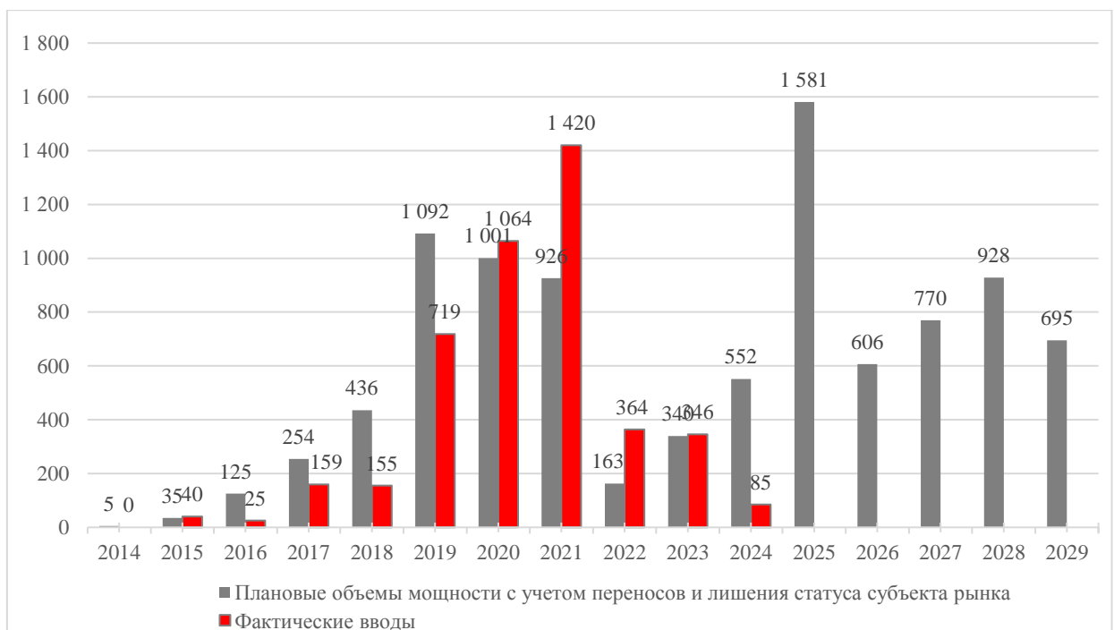
Рис. 2 «Плановые и фактические показатели ввода мощности (с учетом переноса даты начала поставки мощности, изменения величины установленной мощности по объектам генерации ВИЭ и изменений, связанных с лишением права участия по ГТП ДПМ ВИЭ), МВт».
