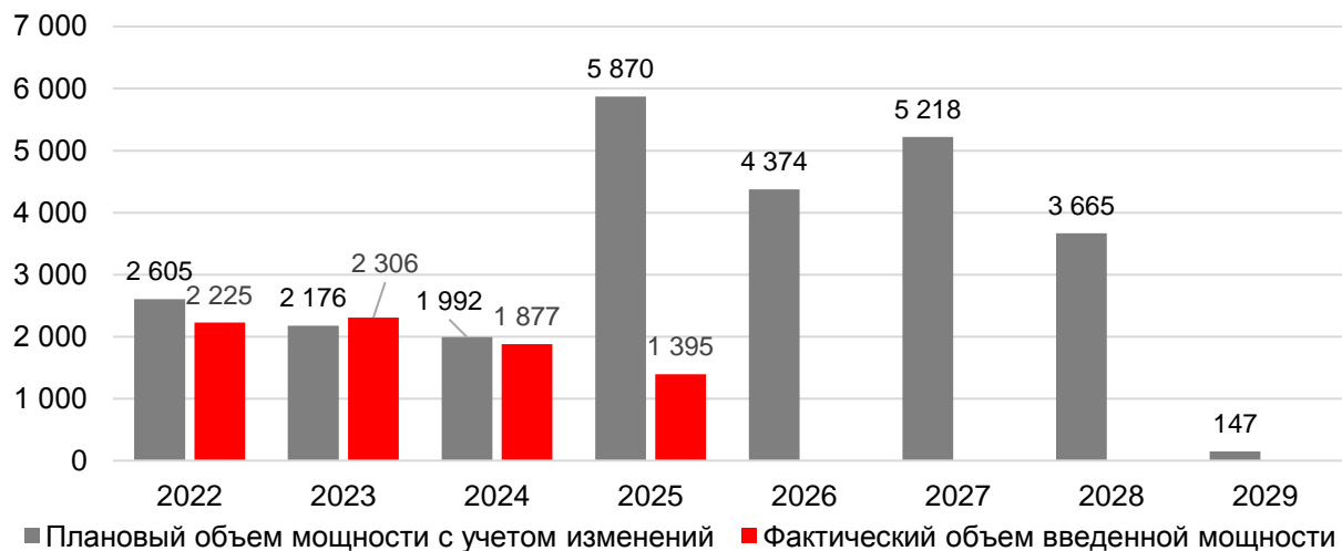
Рис. 2 Плановый (с учетом изменений состава и параметров объектов) и фактический объем мощности модернизируемых объектов генерации, МВт.
