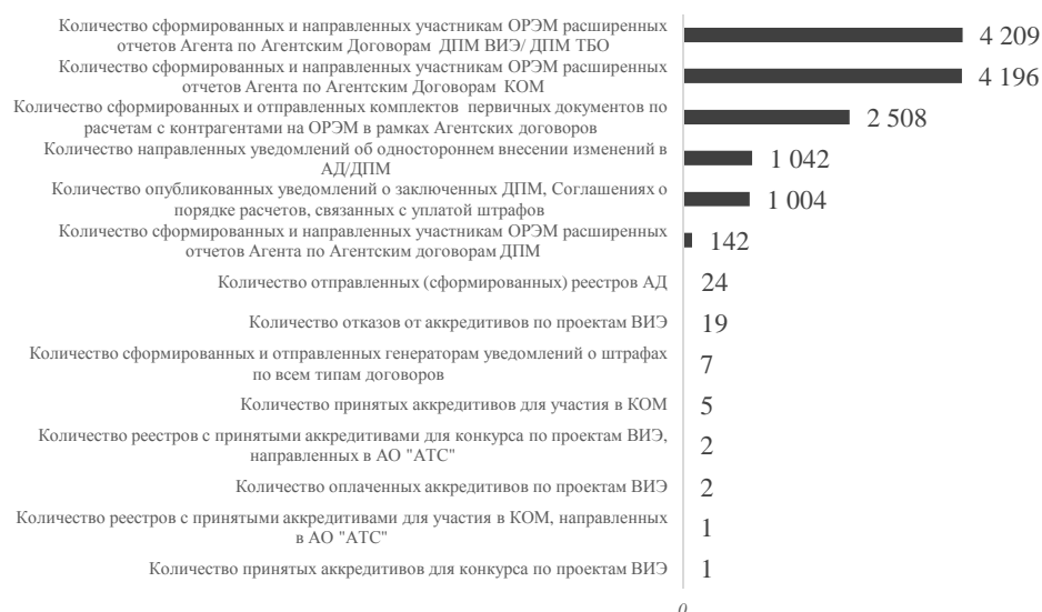
Рис. 6. Функции Агента
