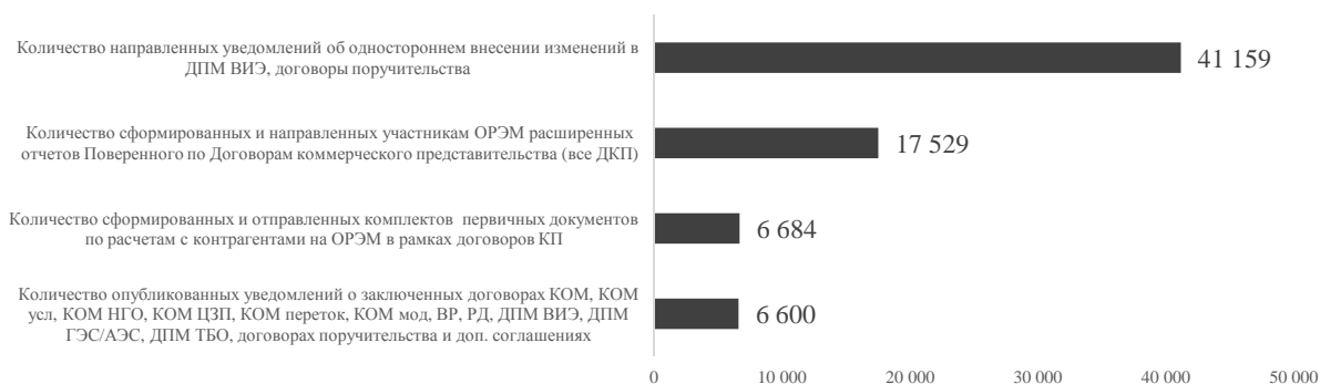
Рис. 8. Функции Поверенного
