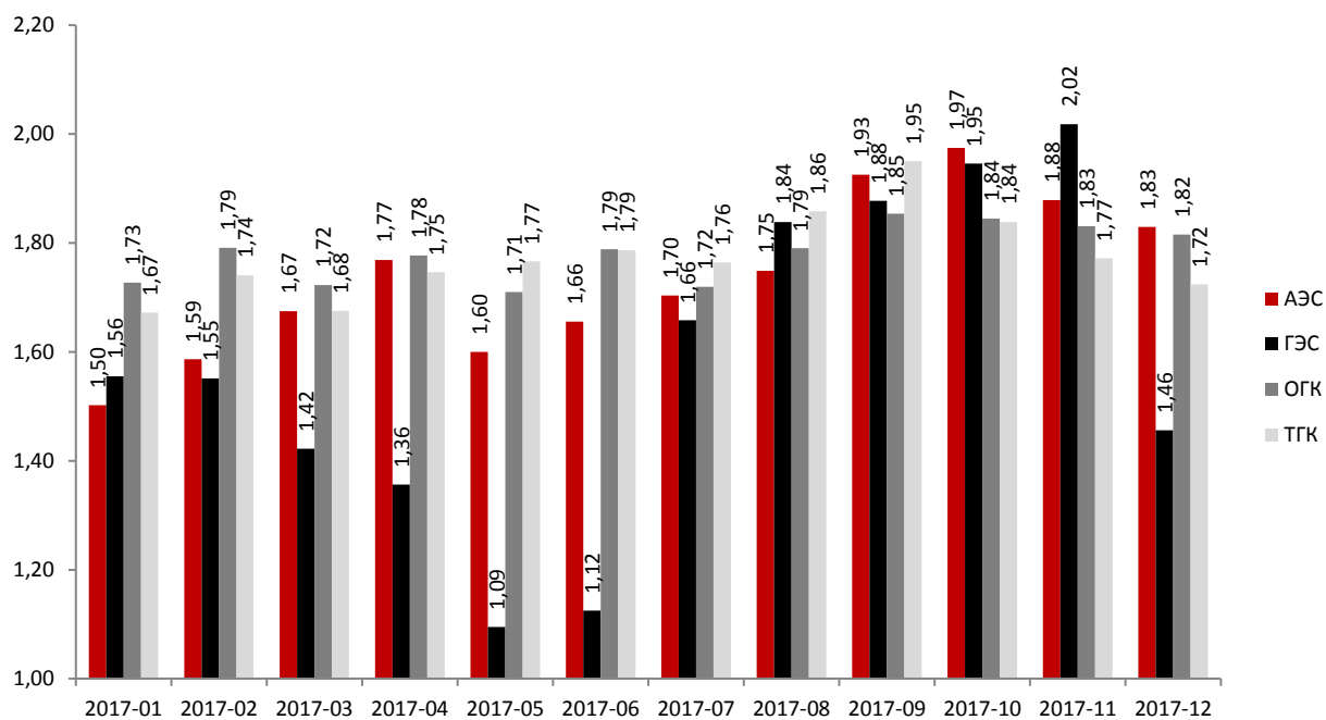
Рис. № 3: Среднеотпускная цена 4 поставщиков электроэнергии за 1 кВтч, с учетом мощности, по типу генерации за 2017 год
